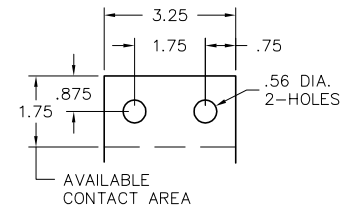
800 A. TERMINAL
