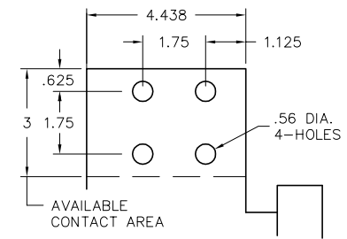
3000 A. TERMINAL
