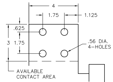
1200-2500 A. TERMINAL
